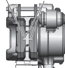
Freno posteriore
