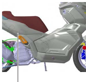
Connettore strumento di diagnosi
